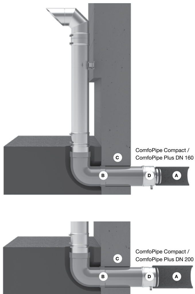
2 ComfoVent 180 Sistem 2 Pod zemljo
